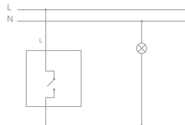
Одноклавишный однополюсный выключатель
