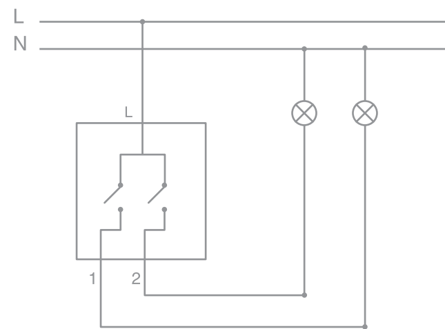
Двухклавишный выключатель
