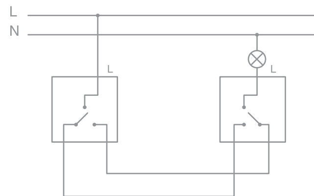
Управление освещением с двух мест
